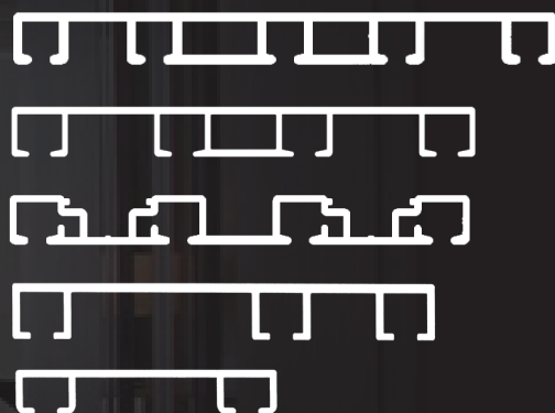
SCALA . SCALE 1:2
